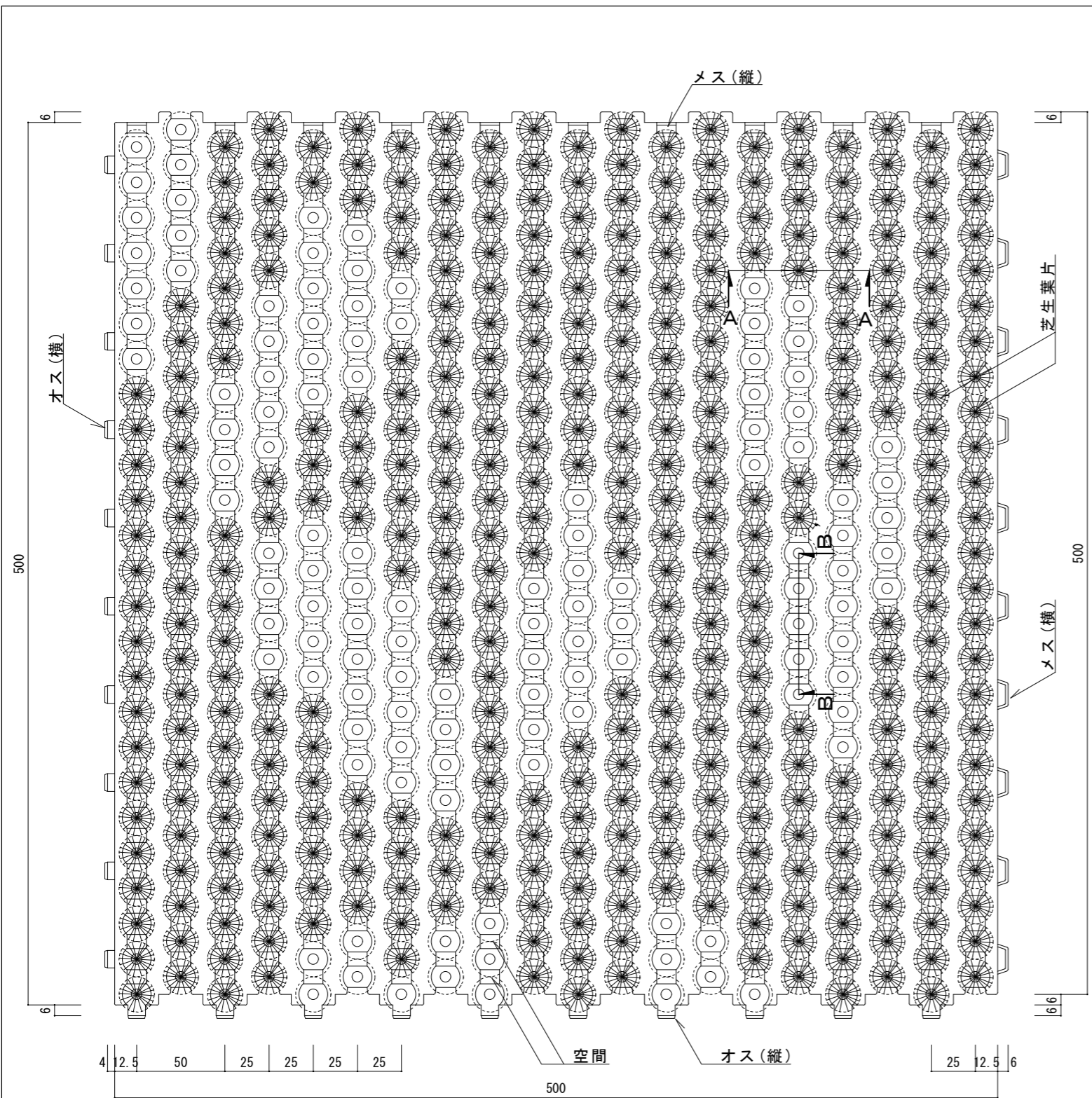
平面図 S=1/3
