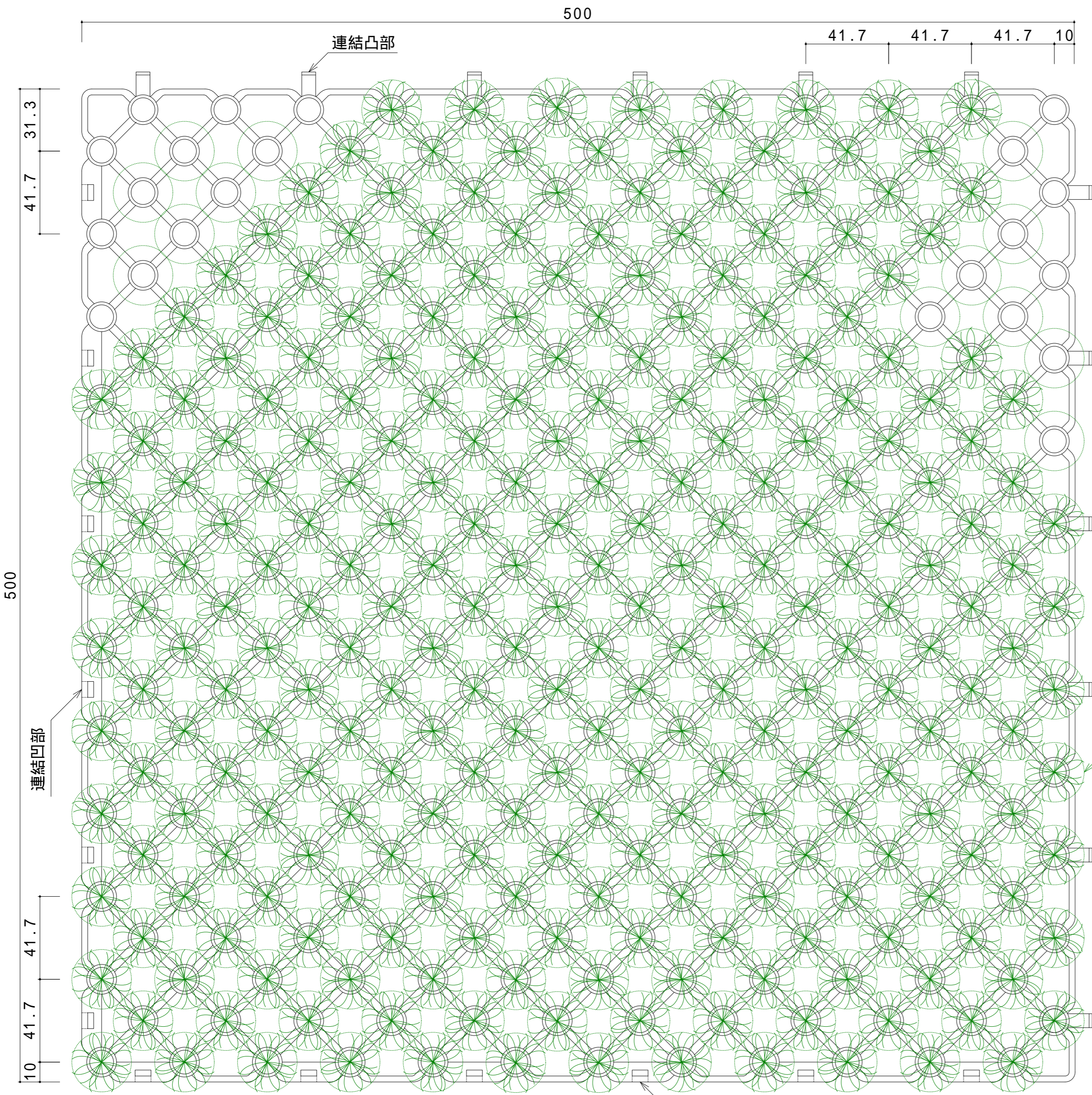
平面図
